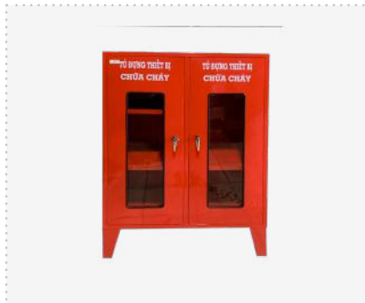
Tủ đựng dụng cụ phá dỡ có chân
