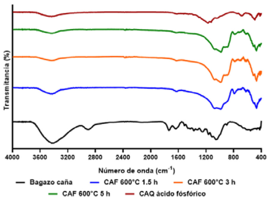
Figura 1. Espectros infrarrojos de los materiales adsorbentes.
