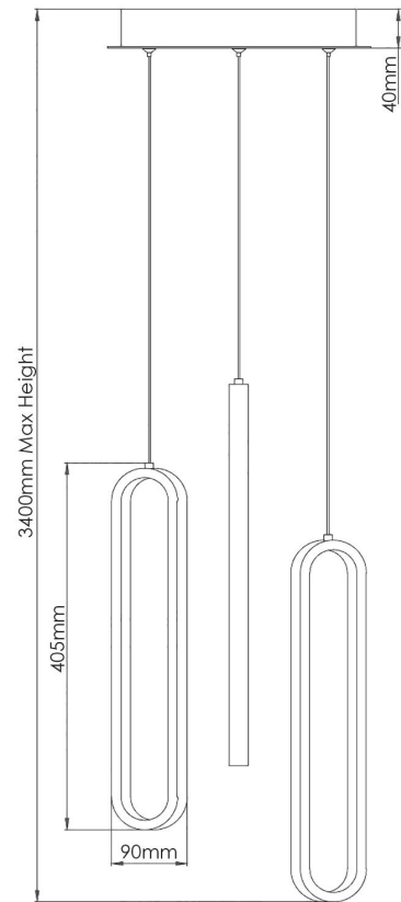
Model: Oval 3 Light Pendant
