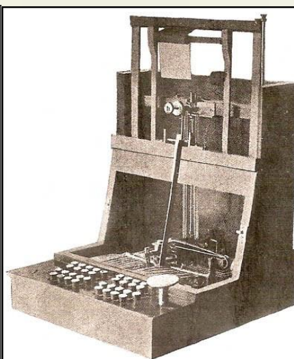
Máquina de escribir de Sholes
