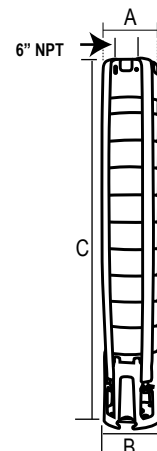
Acoplamiento NEMA 10" Fig. 2
