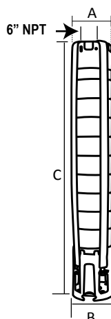
Acoplamiento NEMA 6" Fig. 1
