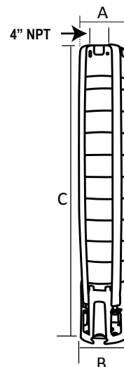
Acoplamiento NEMA 6" Fig. 2
