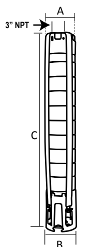
Acoplamiento NEMA 6" Fig. 1
