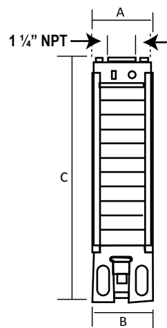
Acoplamiento NEMA 4"
