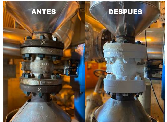
AISLACION TERMICA DE VALVULAS Y PUENTES TERMICOS
