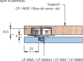
Vue en coupe montrant une installation type (1:2)
