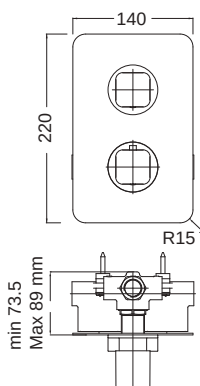
750033NQSL 2 ή 3 εξόδων
