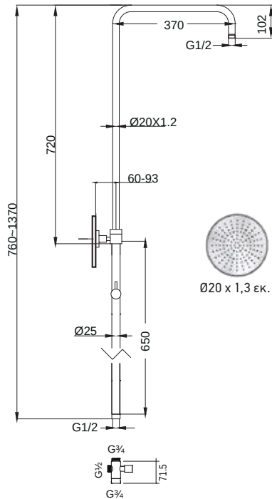
κολώνα ρυθμιζόμενου ύψους
