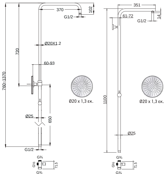
κολώνα ρυθμιζόμενου ύψους
