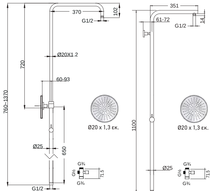
κολώνα ρυθμιζόμενου ύψους
