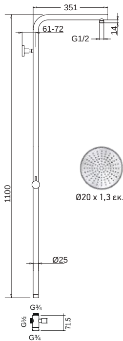
κολώνα σταθερού ύψους
