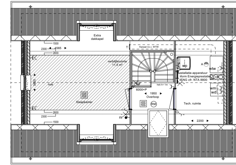
2e verdieping
