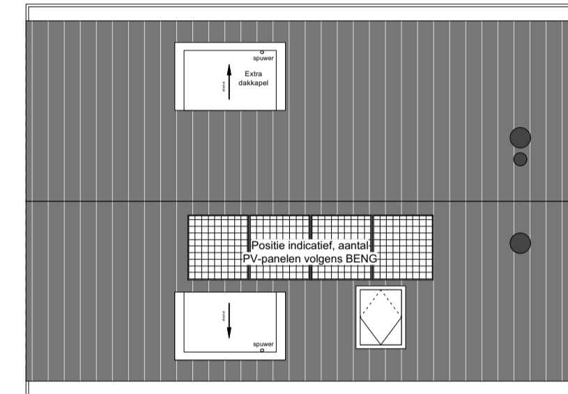
Dakaanzicht
