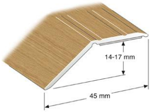
Nivålist Eik nr. 179. Selvkl. 10-16 mm Nivålist Eik nr. 179. Selvkl. 10-16 mm Nivålist Eik nr. 179. Selvkl. 10-16 mm
