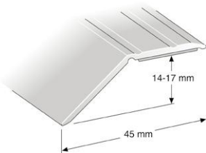
Nivålist Sølv nr. 193. Selvkl. 10-16 mm Nivålist Sølv nr. 193. Selvkl. 10-16 mm
