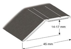
Nivålist Grafitt nr. 269. Selvkl. 10-16 mm Nivålist Grafitt nr. 269. Selvkl. 10-16 mm
