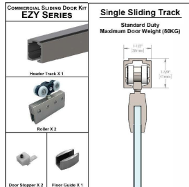
EZY1SD Single Sliding Door Kit
