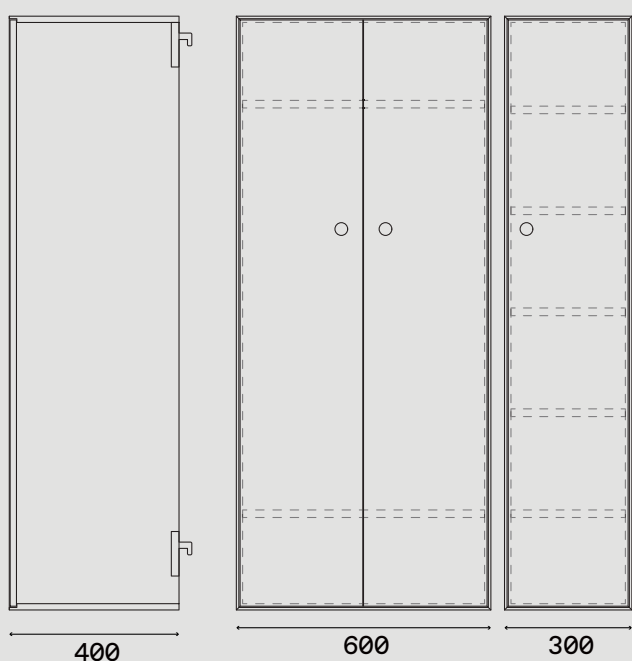
Schrankmodule Doppeltür
