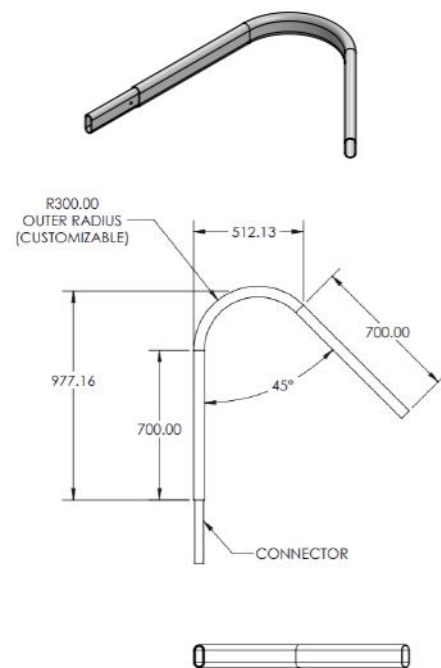
CHUTE END
