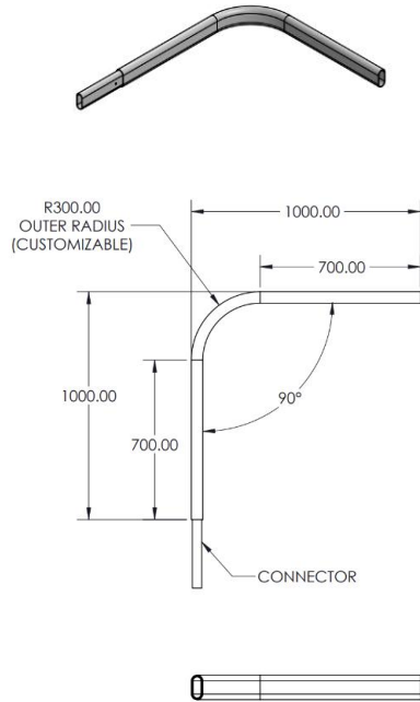
90° BEND
