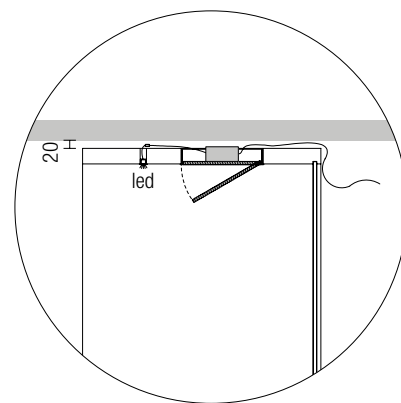
Trasformatore incassato SCATOLA ELETTIFICATA INCASSATA CON SPORTELLINO ISPEZIONABILE
