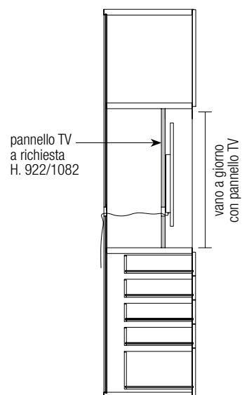
vano a giorno con cassetteria esterna, ante e pannello TV
