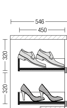
cassettera base - standard con vassoio portascarpe estraibile
