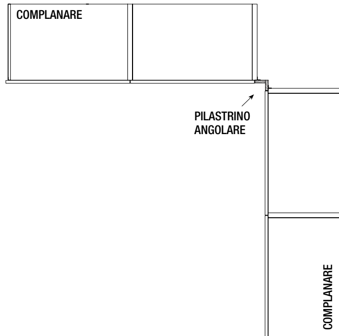
ANGOLO NON USUFRUIBILE COMPLANARE/COMPLANARE
