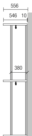
SPALLE TELAIO ALLUMINIO SENZA VETRO
