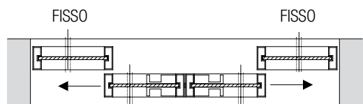
2 pannelli scorrevoli + 2 pannelli fissi binario 2 vie
