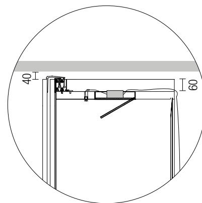
Trasformatore incassato OPTIONAL SCATOLA ELETTTRIFICATA INCASSATA CON SPORTELLINO ISPEZIONABILE 60W USA / ITA 80W USA / ITA
