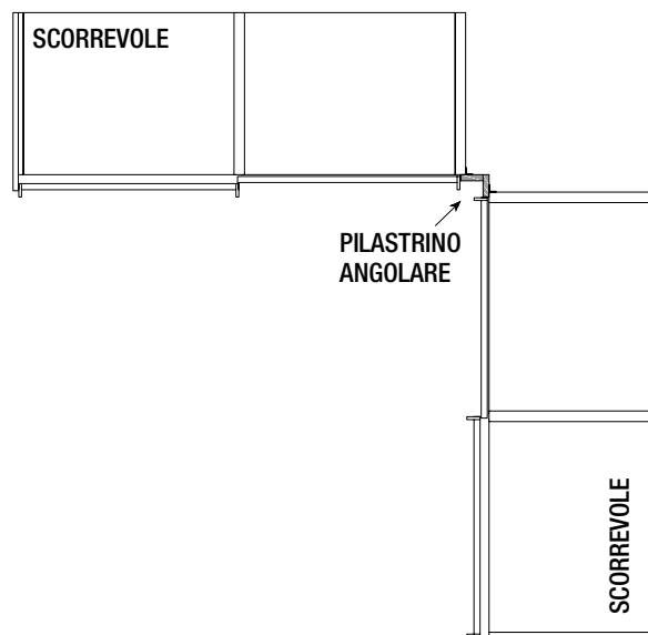
ANGOLO NON USUFRUIBILE SCORREVOLE/SCORREVOLE
