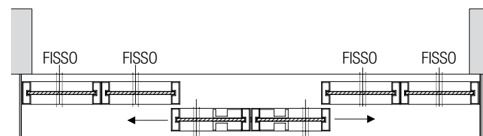
2 pannelli scorrevoli + 4 pannelli fissi binario 2 vie
