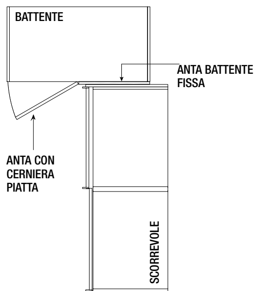
COMBINAZIONI ANGOLO BATTENTE/SCORREVOLE
