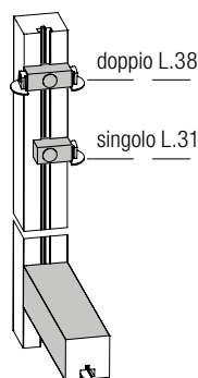
TELAIO CENTRALE SENZA VETRO
