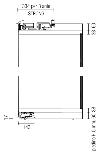
Complanare a nr. 3 ante per mod. 922-1082
