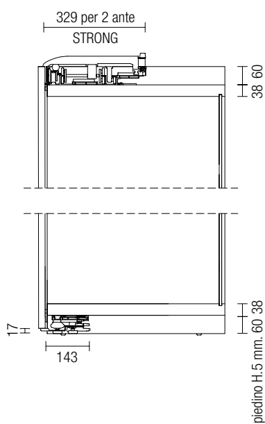
Complanare a nr. 2 ante per mod. 1402
