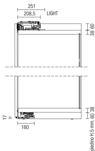
Complanare a nr. 2 ante per mod. 922-1082
