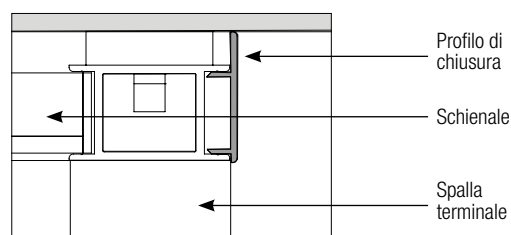
Schienali legno Sp.19mm.
