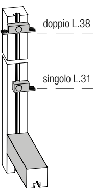
TELAIO CENTRALE SENZA VETRO
