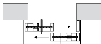
2 pannelli scorrevoli binario 2 vie
