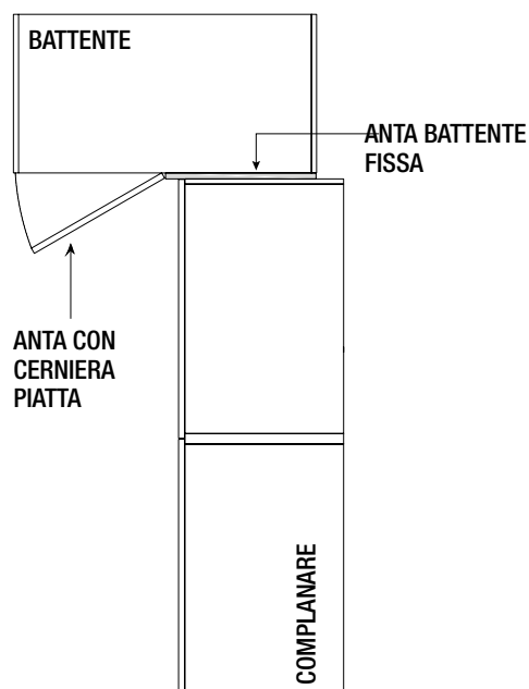
COMBINAZIONI ANGOLO BATTENTE/COMPLANARE
