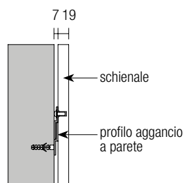
Pannelli legno Sp.19mm.
