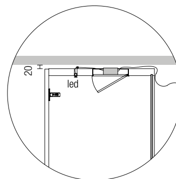
Trasformatore incassato OPTIONAL SCATOLA ELETTRIFICATA INCASSATA CON SPORTELLINO ISPEZIONABILE 60W USA / ITA 80W USA / ITA
