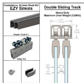
EZY1HDDD (Lourd) Kit de porte coulissante double
