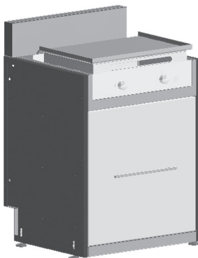
Module plancha gaz - 67 cm Mini crédence de 16 cm
