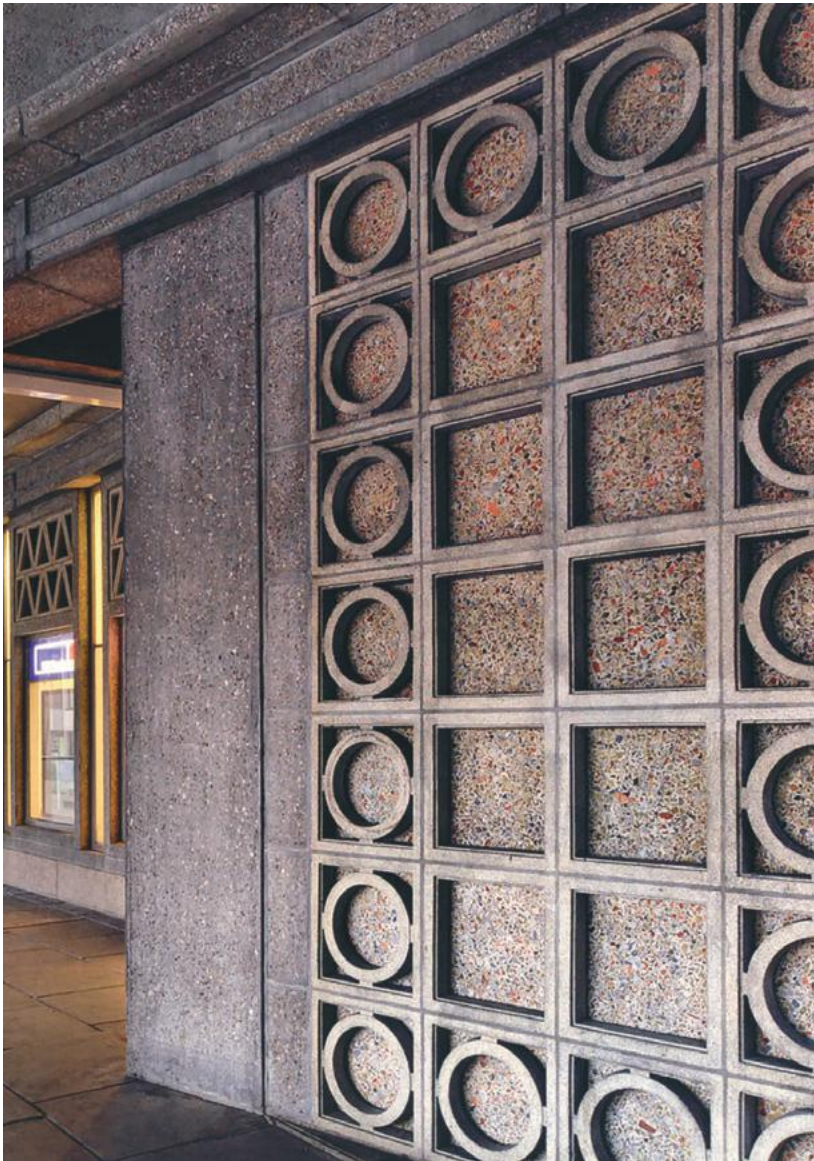
Station Enschede, detail in oostfaçade waarin toeslagstoffen goed te zien zijn
