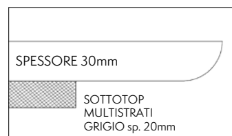
SEZIONE TOP - MATERICO
