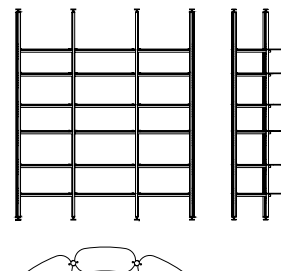
G - 2 MODULI SOFFITTO 248 x 34 x H < 300* CM 98" x 13" x H < 94,5"* REGOLABILE \pm 15 CM
