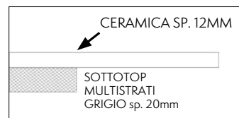
SEZIONE TOP - CERAMICA
