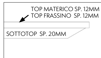
SEZIONE TOP - MATERICO - FRASSINO
