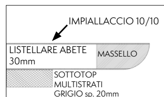
SEZIONE TOP - LEGNO MASSELLATO
