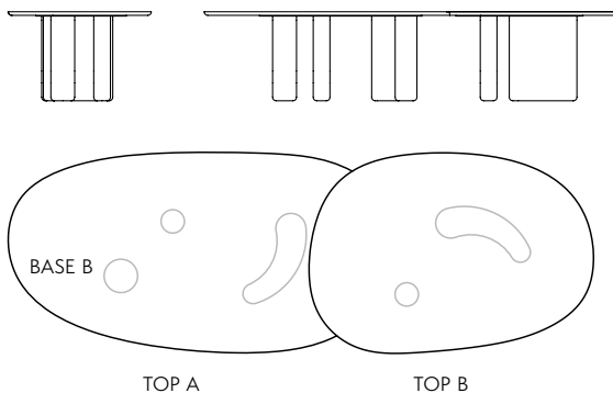
SEZIONE TOP - MATERICO
