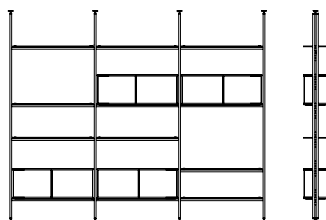
H - 3 MODULI SOFFITTO 370 x 34 x H < 300* CM 145.5" x 13" x H < 94,5"* REGOLABILE \pm 15 CM
