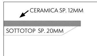
SEZIONE TOP - CERAMICA
