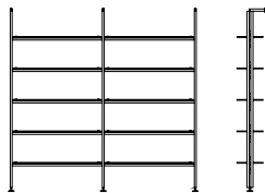
B - 2 MODULI A PARETE 249 x 36.5 x H 240* CM 98" x 14,3" x H 94,5"* * REGOLABILE \pm 7.5 CM
