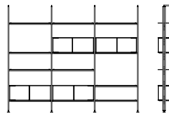
D - 3 MODULI A PARETE 128 x 36.5 x H 240* CM 50,4" x 14,3" x H 94,5"* * REGOLABILE \pm 7.5 CM
