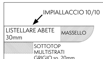
SEZIONE TOP - LEGNO MASSELLATO
