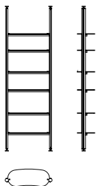
E - 1 MODULO SOFFITTO 94 x 34 x H < 300* CM 37" x 13" x H < 94,5"* REGOLABILE \pm 15 CM
