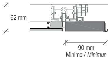
Fascia di tamponamento terminale Terminal filler
