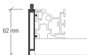
Chiusura laterale INIZIALE INITIAL side closure
