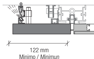
Fascia di tamponamento con LED iniziale Initial filler with LED
