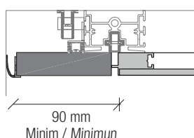
Fascia di tamponamento iniziale Initial filler
