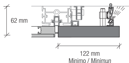
Fascia di tamponamento con LED terminale Terminal filler with LED
