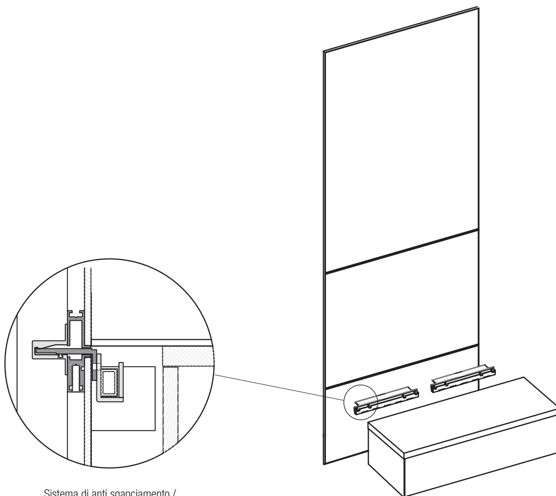
Sistema di anti sganciamento / System of anti release
