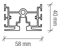
Montante centrale Central upright
