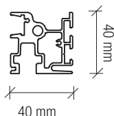
Montante iniziale Initial upright
