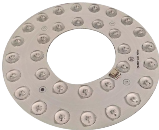
REPUESTO LED VENTILADOR SF CLAVE S00833 S00834
