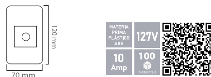
TAPA CONEXIÓN TV DC-013/B CLAVE S00914
