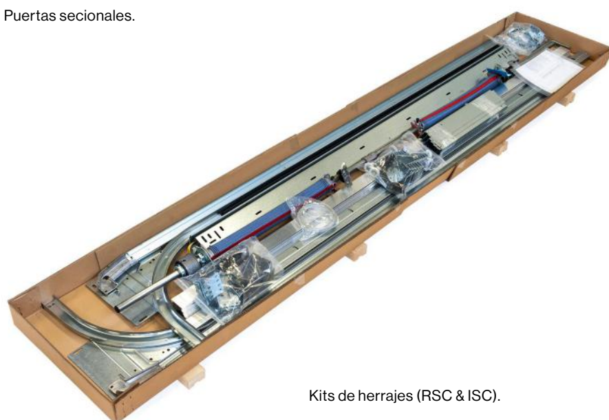
Puertas seccionales.
