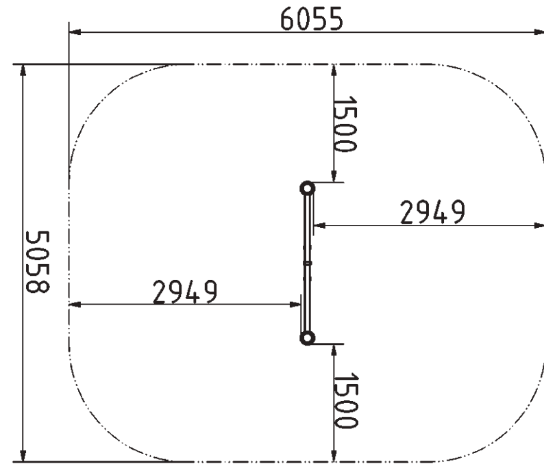
Felülnézet
