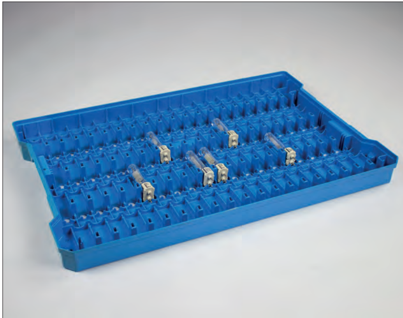
Standaard productdrager met lampjes van Signify (voorheen Philips). De vorm van de buitenkant ligt vast, net als dat het stapelbaar is op andere productdragers. Alleen het binnenwerk is klantspecifiek.
