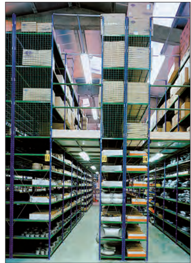
Een Prospace+ stelling met tussenvloer. Deze stelling is 4,5 m hoog en heeft 11 opslag niveaus die dankzij gangpaden gemakkelijk bereikbaar zijn.
