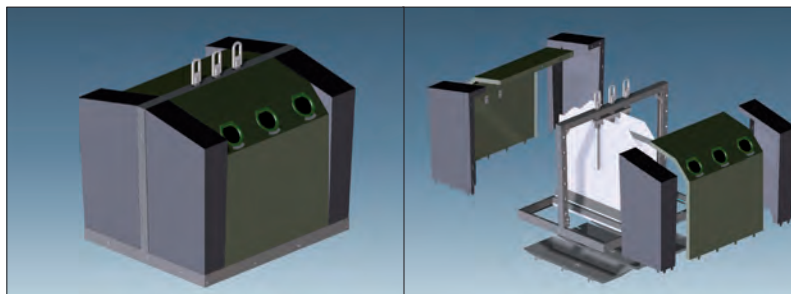
De openingen voor de glas en/of papier inwerpen zijn strak afgewerkt met een kunststof of RVS inwerpopening met rubber of RVS klep.
