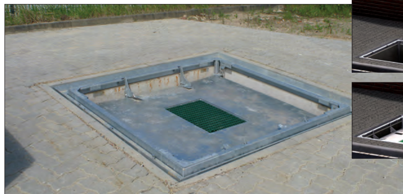
Veiligheidsvloer, alternatief voor het veiligheidshek.
