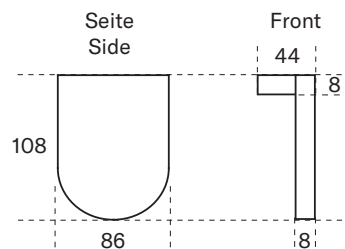
Trägermasse / Fitting dimensions mm
