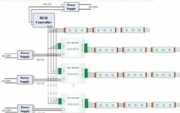
DIAGRAMA DE CONEXIÓN RGB
