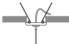
Sujeción techo flotante sin florón (fuente remota sobre el techo)
