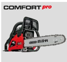
COMFORT pro 6240, 40 cm prowadnica 2-suw / 40,1 cm 3 / 1,5 kW. Łańcuch 3/8" HM, waga 4,6 kg. Nr Artykułu: 127392
