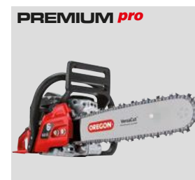
PREMIUM pro 6656 JEDNOSTKA GŁ. 2-suw / 55,5 cm 3 / 2,4 kW. System antywibracyjny, easy start, primer, boczny naciąg łańcucha, regulacja przepływu oleju, podgrzewanie powietrza do pracy zimą. Z zaworem dekompresyjnym. Waga 5,6 kg Nr Artykułu: 127564
