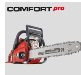
COMFORT pro 6442, 40 cm prowadnica 2-suw / 41,9 cm 3 / 1,7 kW. Łańcuch 3/8" HM, waga 4,8 kg. Podgrzewanie powietrza do pracy zimą. Nr Artykułu: 127430
