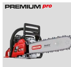
PREMIUM pro 6651 JEDNOSTKA GŁ. 2-suw / 50,9 cm 3 / 2,2 kW. System antywibracyjny, easy start, primer, boczny naciąg łańcucha, regulacja przepływu oleju, podgrzewanie powietrza do pracy zimą. Z zaworem dekompresyjnym. Waga 5,6 kg. Nr Artykułu: 127564
