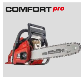
COMFORT pro 6436, 35 cm prowadnica 2-suw / 35,2 cm 3 / 1,5 kW. Łańcuch 3/8" HM, waga 4,8 kg. Podgrzewanie powietrza do pracy zimą. Nr Artykułu: 127429
