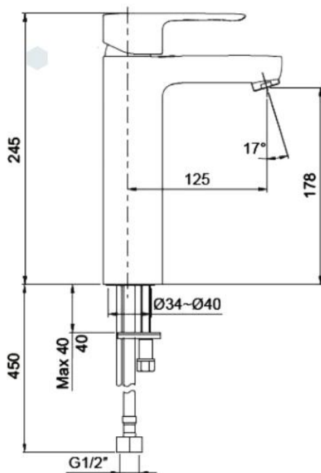
K-5241T-4-CP
