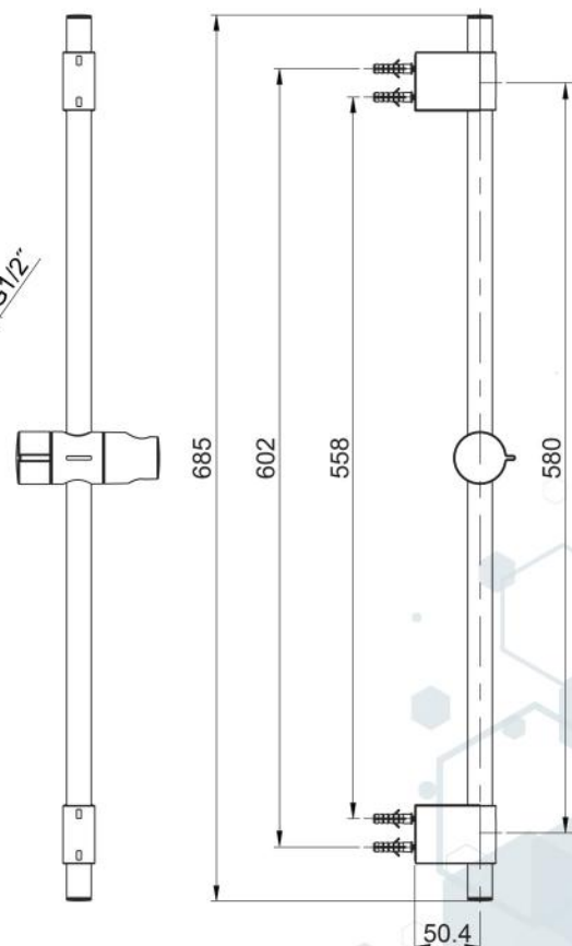
Slide bar
