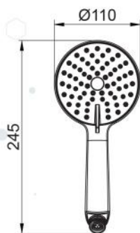
Handshower
