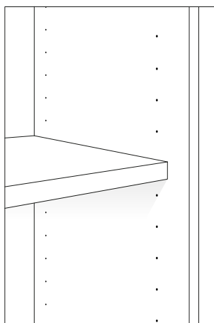
Standard drilling, pitch 96 mm along the entire height of the side panel Foratura standard, passo mm. 96 lungo tutta l'altezza del fianco
