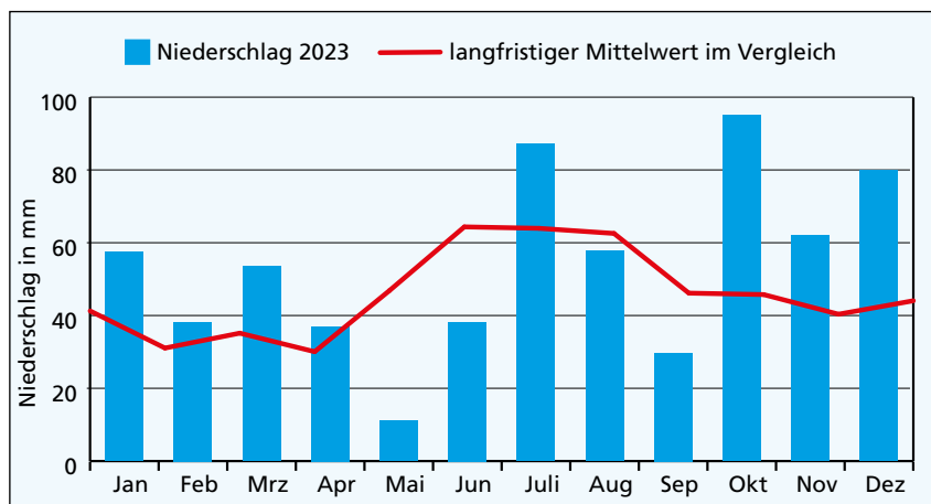
Abbildung 1: Jahresüberblick Niederschlagsmenge Gülzow 2023
