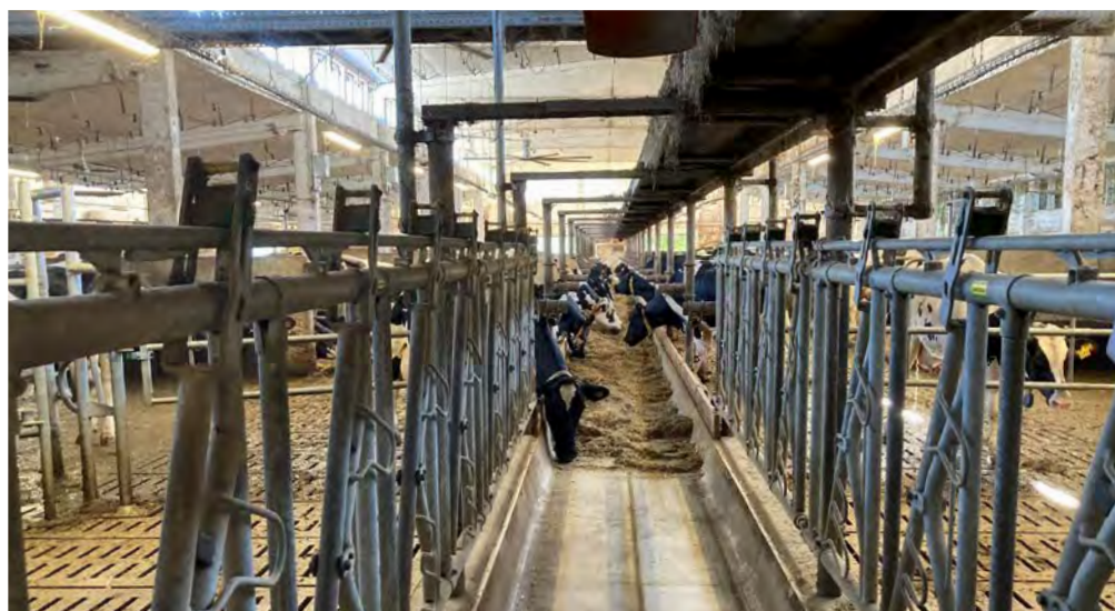
Abbildung 2: Überkopf- Bandfütterungssystem in Altbestandsanlagen
