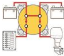
Omskifter: Combine batteries
