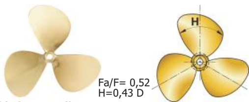
3-bladet propeller, Type P3C (Passer til hurtige både)
