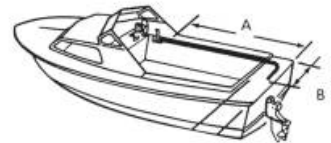
Båd med indenbords motor og drev.
