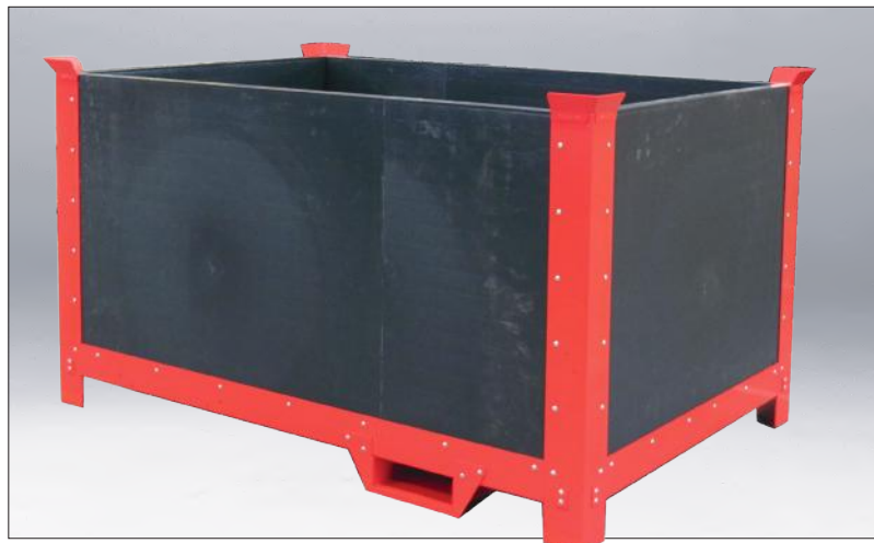
„Stiller“ Auffangbehälter für Blechreste. Ein Rahmen aus Stahl verkleidet mit Hohlkammerplatten aus Kunststoff. Entworfen und gefertigt für Volkswagen.
