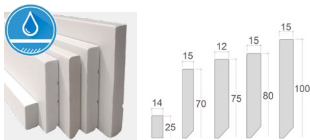
RODAPIÉS ESPUMADOS 100% resistentes al agua. Fabricados con planchas extrusionadas rígidas de PVC expandido.
