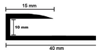
PERFIL U Perfil de aluminio para embutir el pavimento, quedando a la vista una pequeña parte del perfil de manera discreta.
