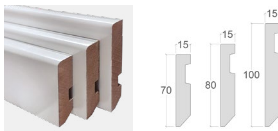
RODAPIÉS DM LACADO BLANCO Canto recto. Resistente a las rayadas.
