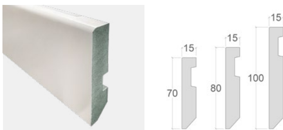
RODAPIÉ DM LACADO BLANCO HIDRÓFUGO Canto recto. Alta resistencia a la humedad.
