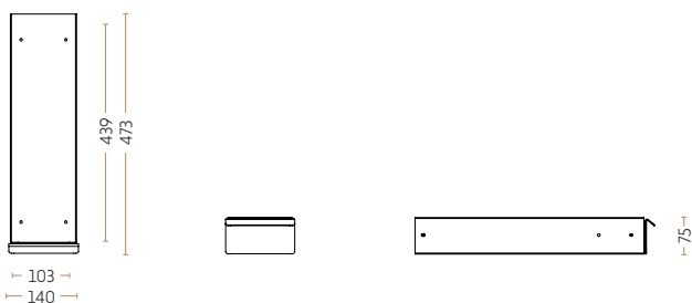
Schublade „Modell narrow Space“ 4058-9005 // 4059-9006 // 4057-9016
