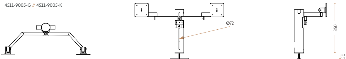
Future Flex für 2 Monitore 4511-9005-G // 4511-9005-K
