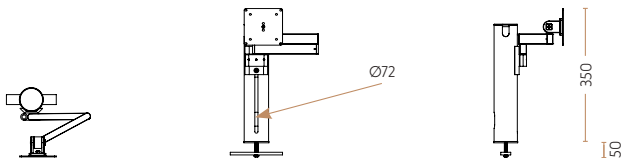
Future Flex für 1 Monitor 4510-9005-G // 4510-9005-K
