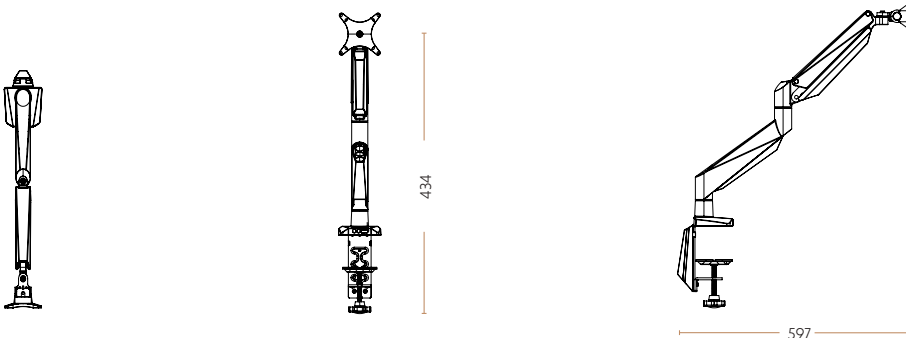
Monitorbefestigung „Monitorarm "Heavy" mit Gasdruchdämpfer" für 1 Monitor 4408-9005
