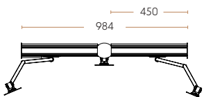
Monitorbefestigung Wings 4160
