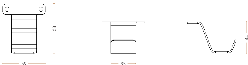
Haken für Tasche 5000-0000-9005 // 5000-0000-9006 // 5000-0000-9016
