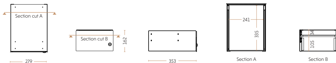
Duo Schublade 4060-2000-9005
