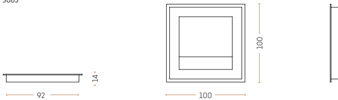
Kabeldurchlass - „Vierkant“ - Klein
