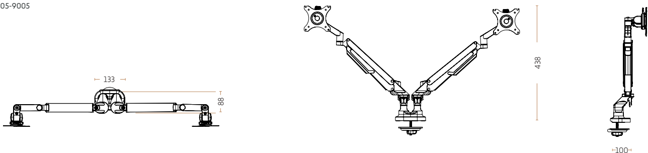
Monitorbefestigung „Monitorarm mit Gasdruckdämpfer“ für 2 Monitore 4405-9005
