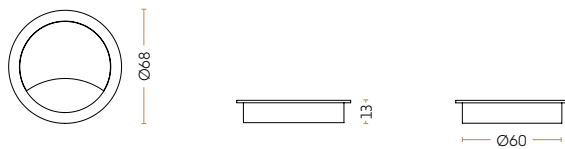
Kabeldurchlass „Rund“ - \text{Ø}60 // Höhe: 13 mm.
