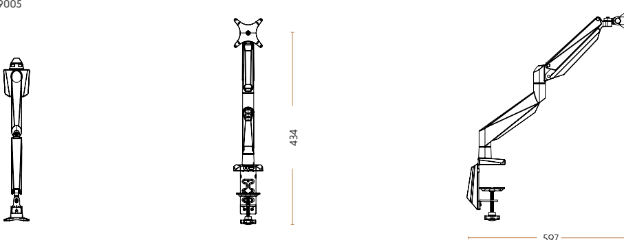
Monitorbefestigung „Monitorarm "Heavy" mit Gasdruckdämpfer" für 1 Monitor 4408-9005
