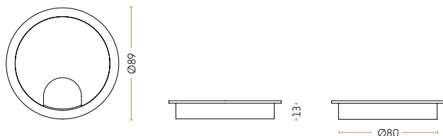
Kabeldurchlass „Rund“ - \text{Ø}80 // Höhe: 13 mm.
