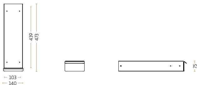
Schublade „Modell narrow Space" 4058-9005 // 4059-9006 // 4057-9016
