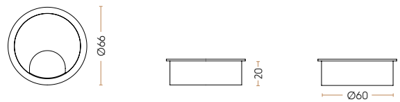
Kabeldurchlass „Rund“ - \text{Ø}60 // Höhe: 20 mm.
