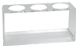
SDHS-3 สำหรับขวดซอส For 12 oz ขนาดช่องใส่ Slot size: Ø7.5 cm (Ø3") W8 x L24 x H9 cm (W3.2" x L9.5" x H3.6")
