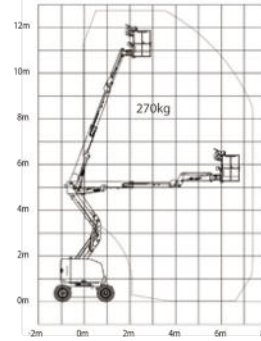
LGMG AR11J
