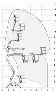
OIL&STEEL OCTOPUS 14
