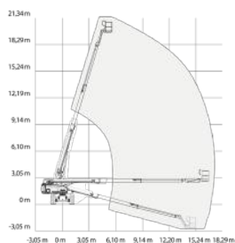
GENIE S-65
