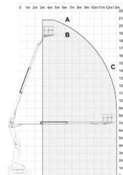
NIFTYLIFT HR21 HYBRID AWD
