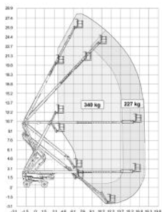
SKYJACK SJ85AJ
