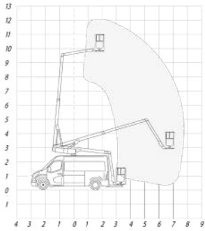
SOGAGE 12VT (Furgoneta)
