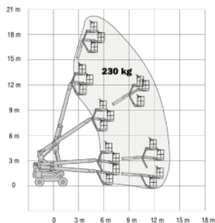
JLG E600JP
