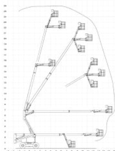
HAULOTTE HA260PX
