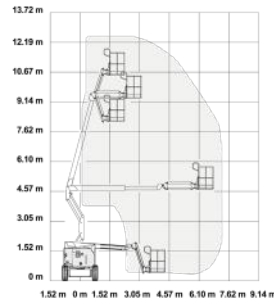
GENIE Z-34/22IC
