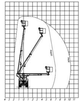
SOCAGE 16T
