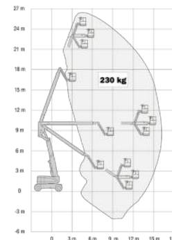
JLG 800AJ
