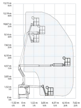
GENIE Z-34/22N
