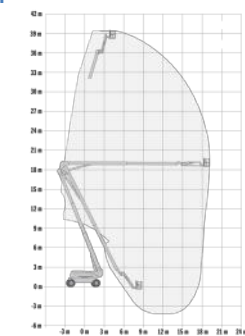
JLG 1250AJP
