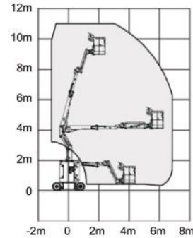
LGMG A09JE
