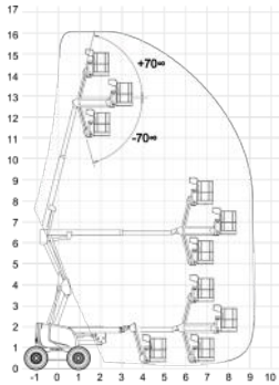
HAULOTTE HA16PX
