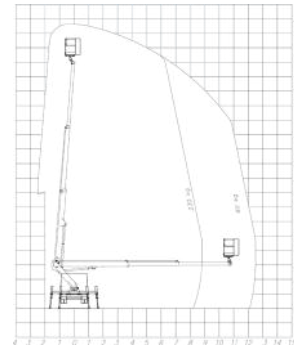
SOCAGE 20T
