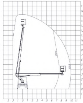
SOCAGE 15T
