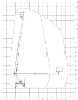
SOCAGE 18T
