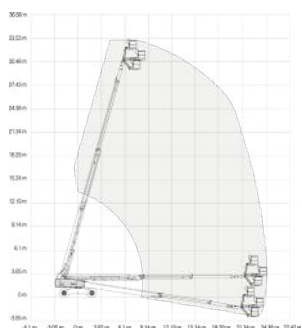
GENIE S-105
