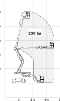
JLG 450AJ
