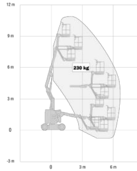
JLG E300AJP
