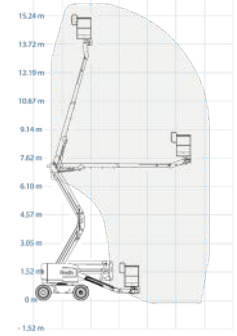
GENIE Z-45/25J
