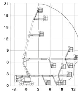
HAULOTTE HA20PX
