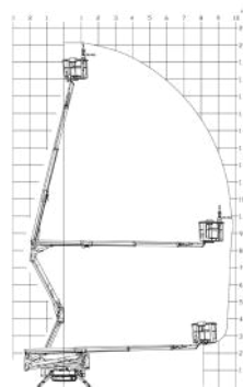
JLG X 20 J PLUS
