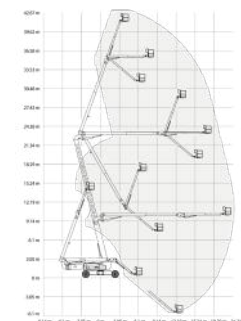
GENIE ZX-135/70
