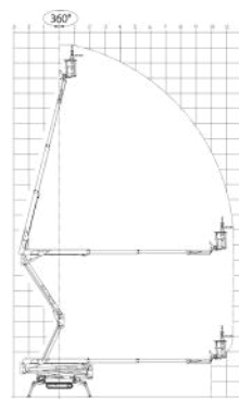
JLG X 23 J
