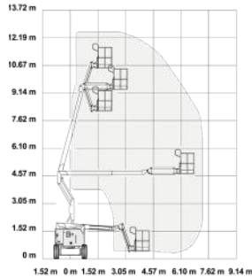
GENIE Z-34/22
