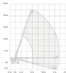
GENIE S-85
