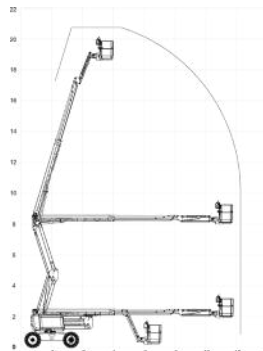
HAULOTTE HA20RTJ
