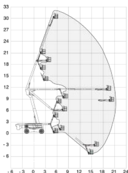
HAULOTTE HA32PX
