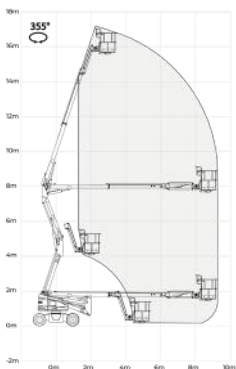
SINOBOOM GTZZ16EJ
