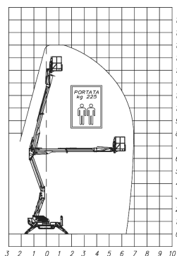
SOCAGE SPJ 315
