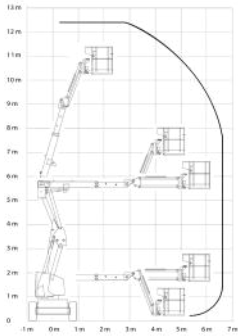
HAULOTTE HA120PX
