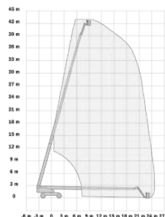
JLG 1350 SJP
