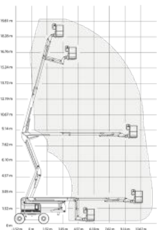
GENIE Z-60/34
