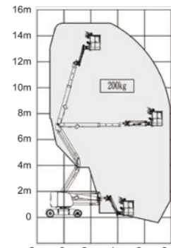
LGMG A13JE
