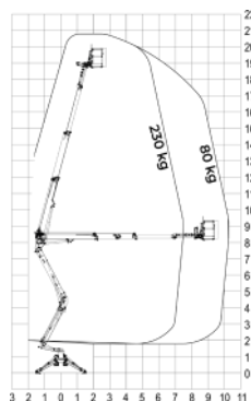
SOCAGE 21 S
