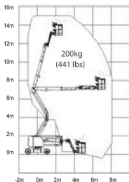
LGMG AR20JE
