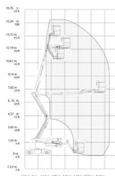
GENIE Z-45/25J DC
