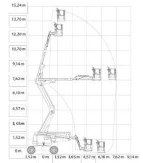
JLG 450AJII
