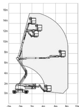
LGMG A14JE
