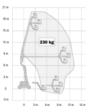
JLG 600AJ
