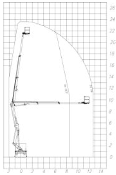
SOGAGE FORSTE 24D
