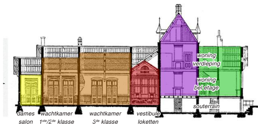
Afb. 4.10: Langsdoorsnede
