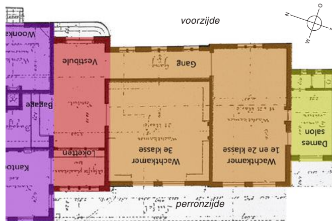
Afb. 4.23: Plattegrond reizigersvleugel
