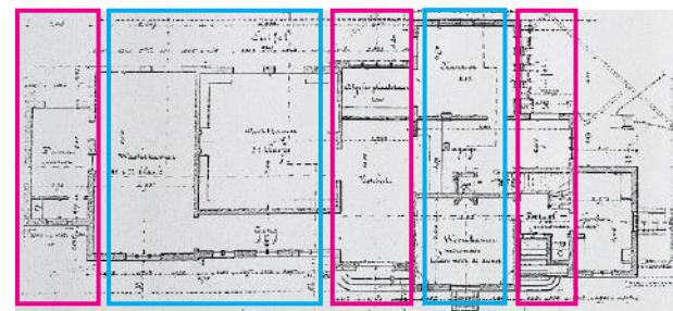
Afb. 1.13: Plattegrond van station Boxmeer. In roze de kenmerken van Rhenen en in blauw de kenmerken van Hemmen
