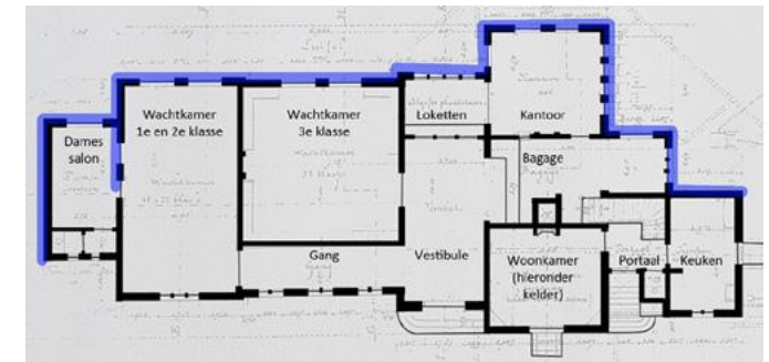
Afb. 4.31: Plattegrond met aanduiding gepleisterde gevels (blauw)
