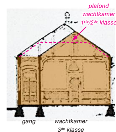
Afb. 4.9: Dwardoorsnede
