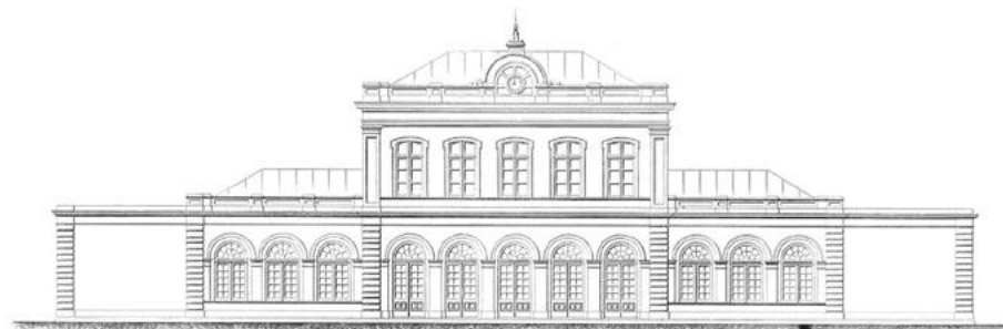
Afb. 1.4: Standaardontwerp derde klasse-station van stations Eerste Staatsaanleg, Waterstaatstijl, architect: K.H. van Brederode
