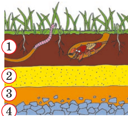
Шари земної поверхні: 1 — ґрунт; 2 — пісок; 3 — глина; 4 — каміння
