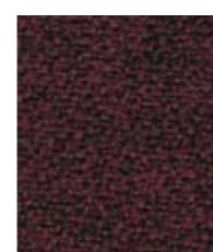
Add AK012
