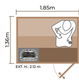
1419RS INT. VOL.: 4.44 m 3 SCA 4.5kW
