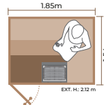
1522LS INT. VOL.: 5.88 m 3 NRN 6.0kW
