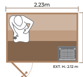
1522LS INT. VOL.: 5.88 m 3 NRN 6.0kW
