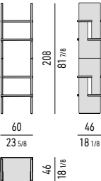
LIBRERIA CM 60X46 H208 - MOD. B BOOKCASE CM 60X46 H208 - MOD. B
