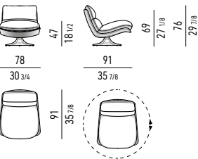
MOVIMENTO GIREVOLE 360° CON RITORNO 360° SWIVEL MOVEMENT WITH RETURN
