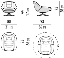
MOVIMENTO GIREVOLE 360   CON RITORNO 360   SWIVEL MOVEMENT WITH RETURN
