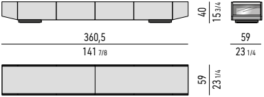
CONTENITORE ORIZZONTALE LIVING CM 360,5X59 H40 LIVING HORIZONTAL SIDEBOARD CM 360,5X59 H40
