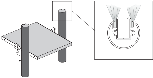
Fissaggio degli elementi al montante /Fixing the elements to the upright
