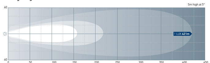
Long Range 011872511
