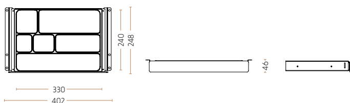
Pennebakke - bred udgaver, med flytbar plastik indsats 4015-9005 // 4016-9006 // 4017-9016
