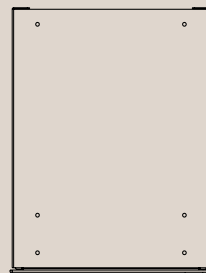
4060-2000-9005 Duo skuffe H: 162 mm. // B: 279 mm. // D: 353 mm. Se mere på side 32-33
