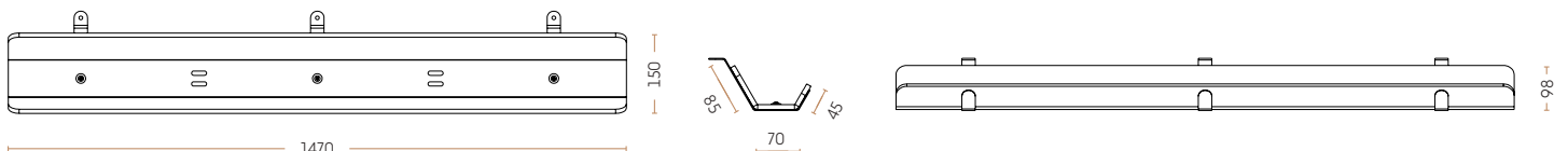
Filtkabelbakke - 147 cm. 6000-0211
