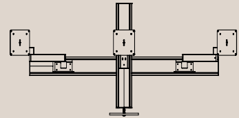
4160 Wings H: 450 mm. // B: 984 mm. // D: 87-120 mm. Se mere på side 68-69
