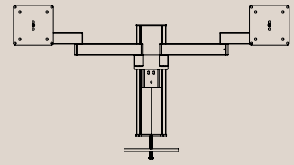
4140-G // 4140-K Skærmsøjle til to skærme. Fås i to versioner Skærmsøjlen: 300 mm. // Forlængerled: 334 mm. Se mere på side 70-71
