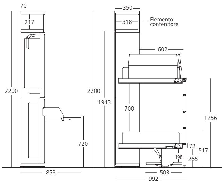
Mobile letto chiuso + scrittoio
