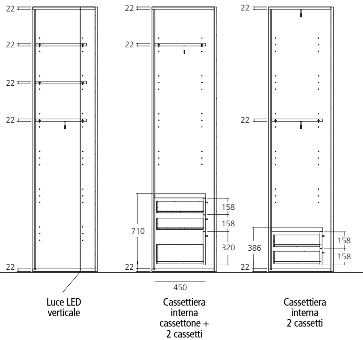
Esempio componibilità colonna
