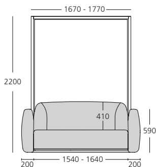
(Fig. 1) divano MINERVA 167 - 177 - due posti
