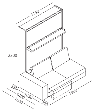
Tango divano 198 (versione sx)
