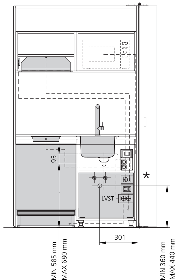
Predisposizione per versione con anta attrezzata dx
