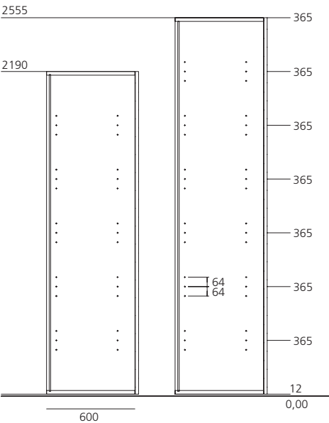
Colonna armadio profondità mm 623
