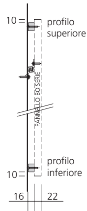
Dettaglio profilo di chiusura superiore
