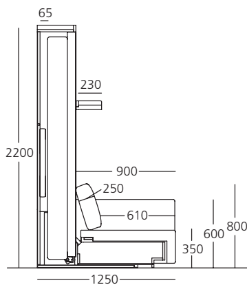
mobile letto chiuso + divano
