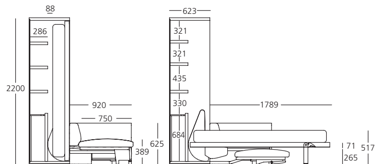
Mobile letto chiuso + Divano
