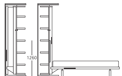
Mobile letto chiuso
