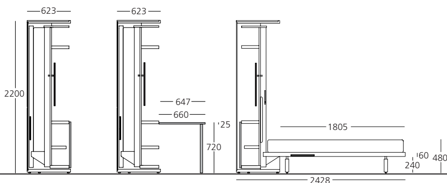
Mobile letto chiuso + tavolo chiuso
