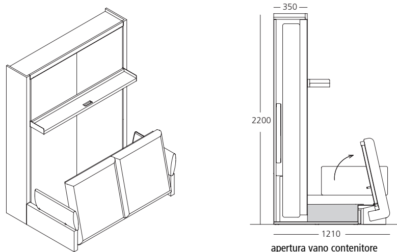
apertura vano contenitore
