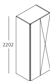
anta con Gola
