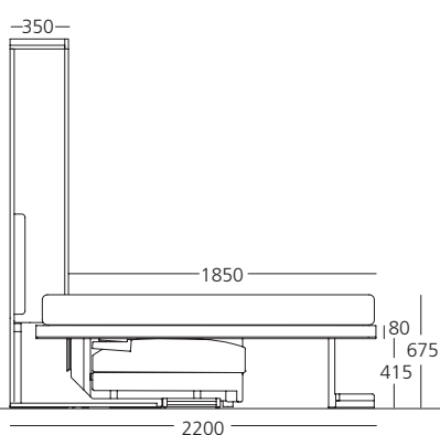
mobile letto aperto
