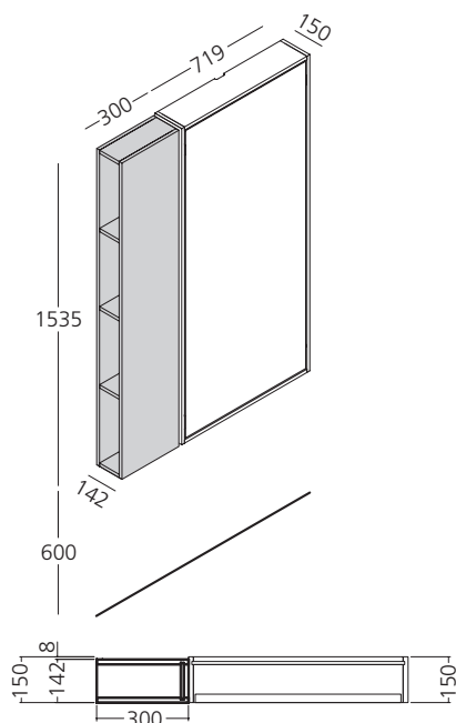
Libreria laterale P. mm 150
