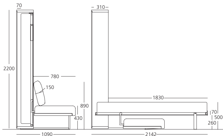
Mobile letto chiuso + Divano
