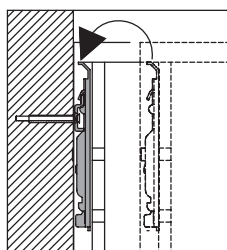
Particolare sezione fissaggio a parete
