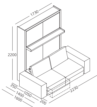
Tango divano 198 (versione sx)
