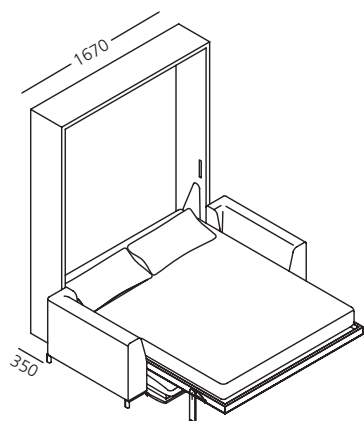
Mobile letto aperto 201 P. 35 - Versione motorizzata Power
