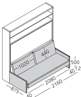
(Fig. 1) Divano con braccioli L mm 40
