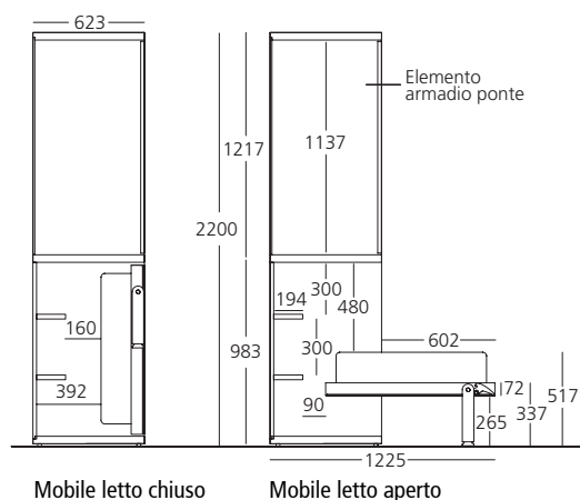
Mobile letto chiuso
