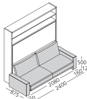
(Fig. 3) Divano versione Next con braccioli L mm 160, seduta divisa, fascia orizzontale sotto seduta
