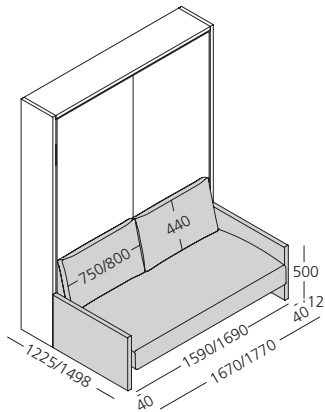
(FIG. 1) DIVANO Versione BASIC divano con braccioli L mm 40
