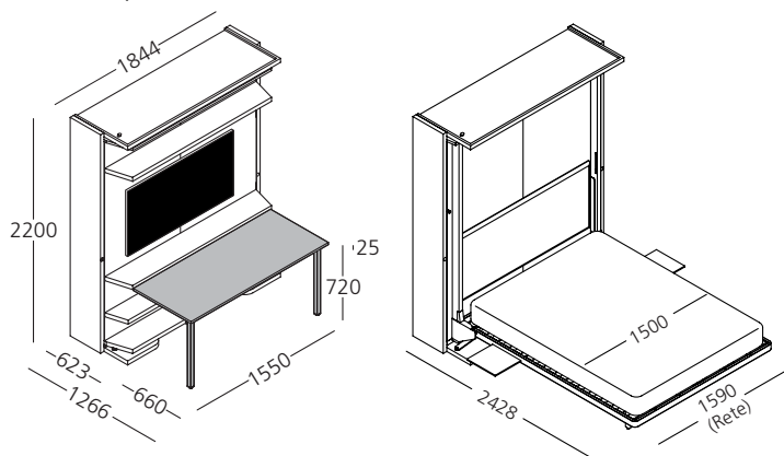
Mobile letto chiuso + tavolo aperto
