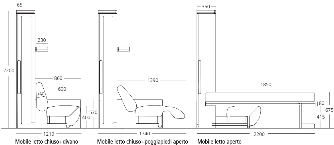
Mobile letto chiuso+divano
