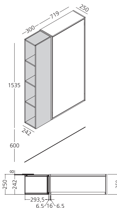
Libreria laterale P. mm 250
