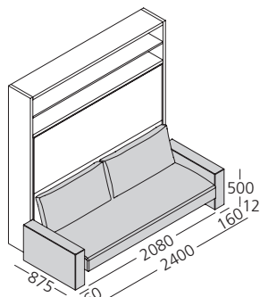
(Fig. 2) Divano con braccioli L mm 160
