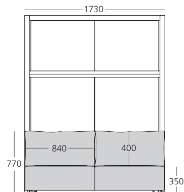
Vista frontale Swing"0"
