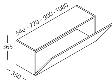
Ribalta con apertura verso il basso
