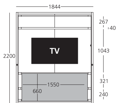
Mensole non spostabili
