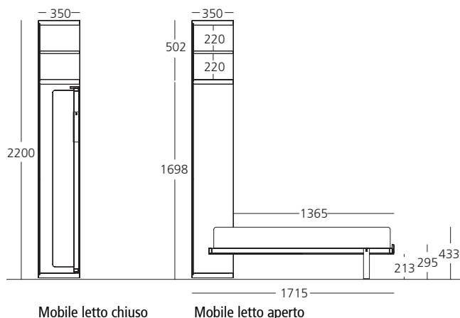
Mobile letto chiuso
