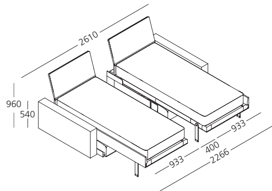
Letti singoli separati - testate reclinabili
