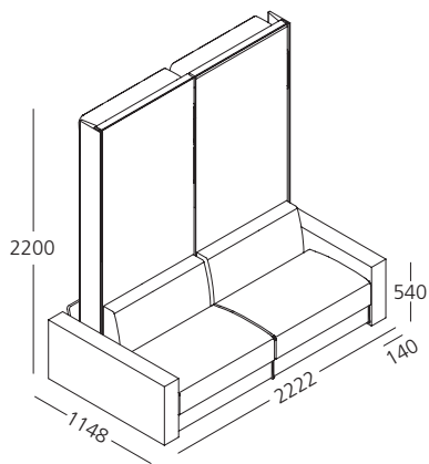
Sistema con letto matrimoniale e divano 2 posti
