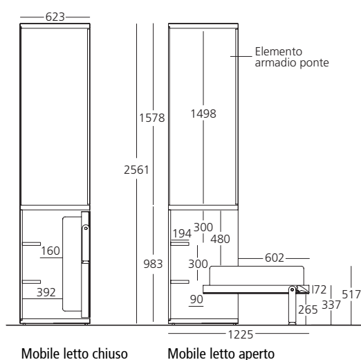
Mobile letto chiuso
