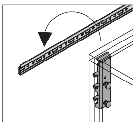
Particolare del sistema di aggancio a parete
