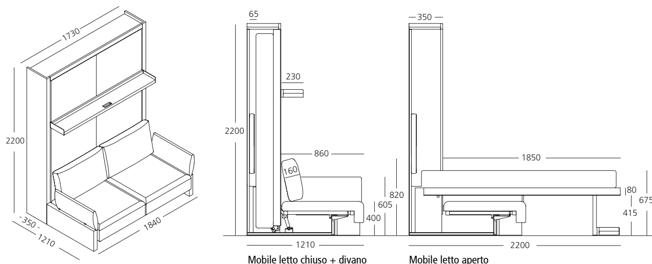
Mobile letto chiuso + divano
