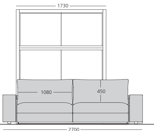
Vista frontale Tango Divano 270
