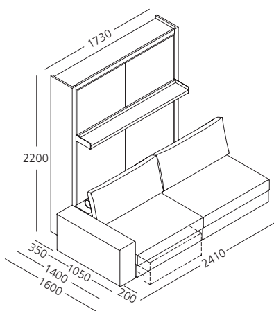
Tango componibile 241 (versione sx)
