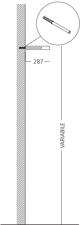
Mensola a parete: sistema di fissaggio a parete
