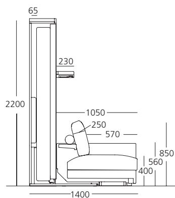
mobile letto chiuso + divano
