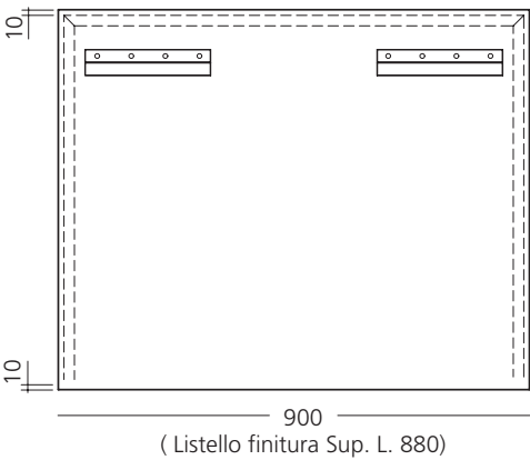
Esempio di combinazione profili di chiusura su tre lati
