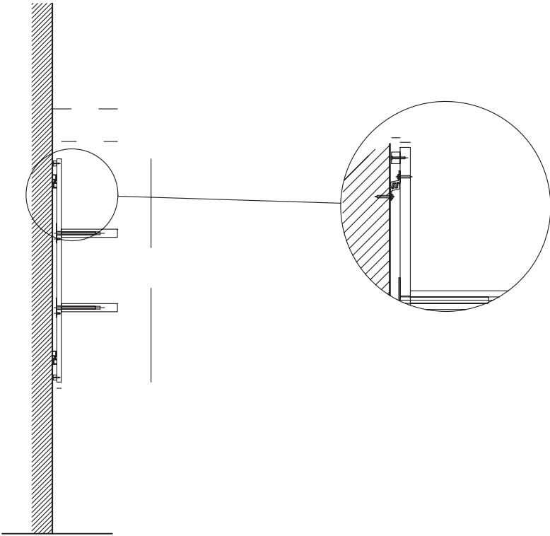
Pannelli modulari sospesi sistema di fissaggio a parete
