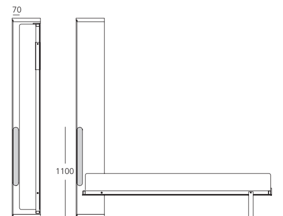
Mobile letto chiuso
