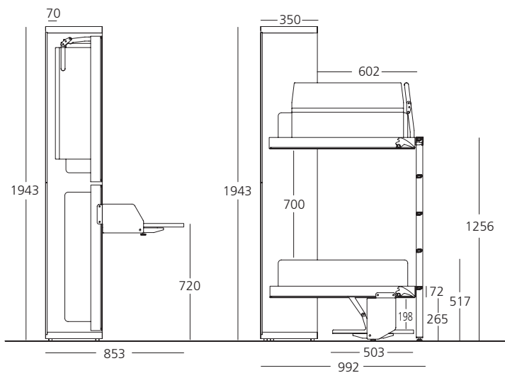
Mobile letto chiuso + scrittoio
