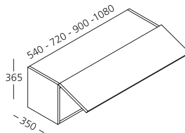
Ribalta con apertura verso l'alto
