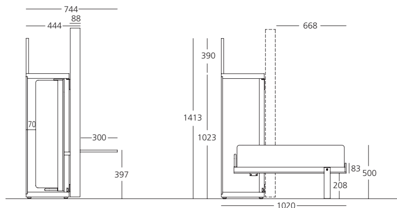
Mobile con letto chiuso
