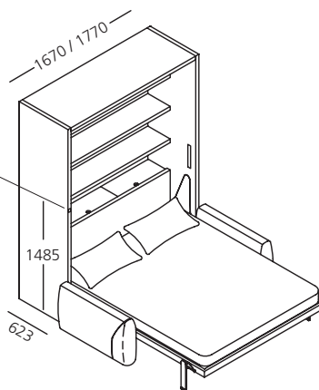
Mobile letto aperto 201 P.62,3 - Versione motorizzata Power
