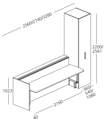
Fianco laterale, Cabrio In, colonna P mm 623 N.B: non è possibile l'affiancamento diretto a colonna in P mm 350
