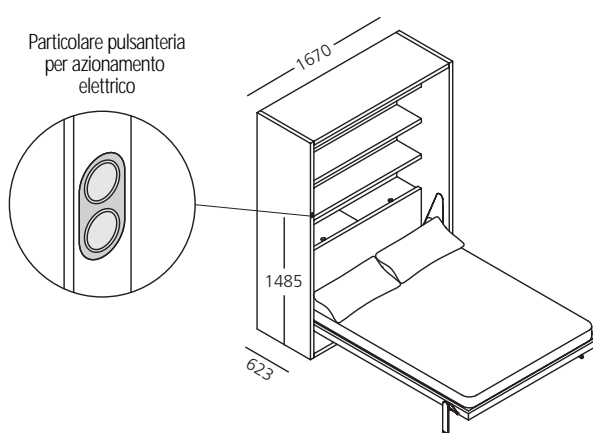
Mobile letto aperto 201 P. 62,3 - Versione motorizzata Power
