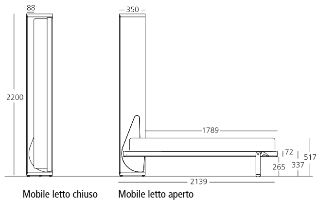
Mobile letto chiuso
