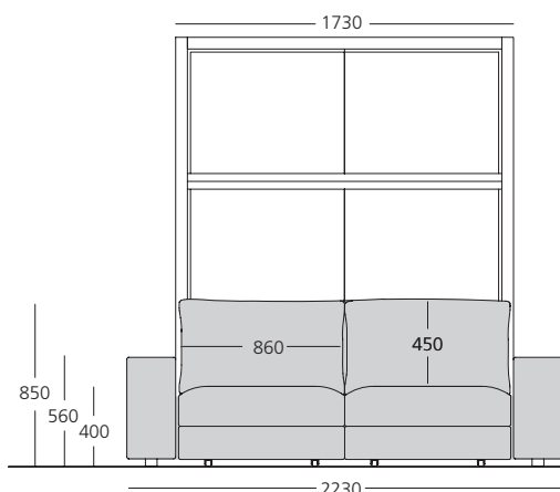
Vista frontale Tango Divano 223
