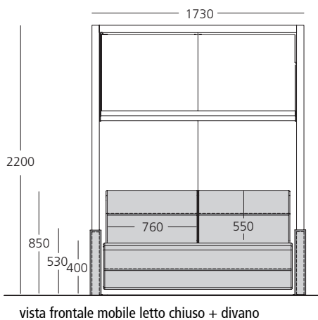
vista frontale mobile letto chiuso + divano
