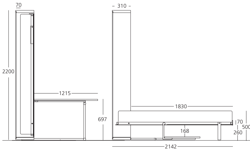
Mobile letto chiuso + Work
