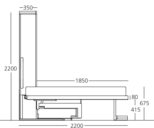
mobile letto aperto
